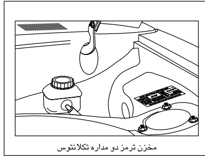
مخزن ترمز دو مداره تک‌لانتوس
